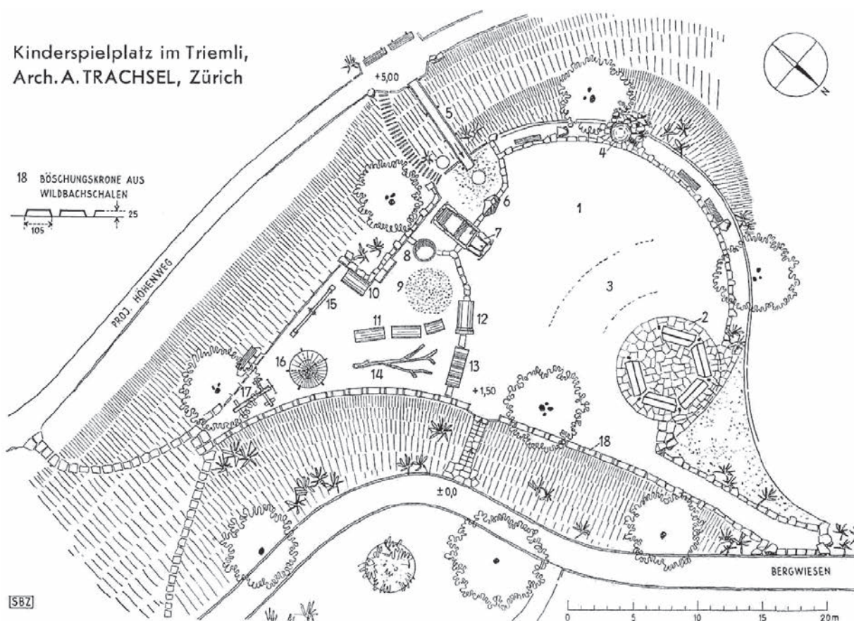
Bild 5. Lageplan 1:500
