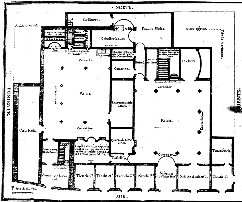
Plano de la planta baja del Palacio Municipal AGI, Mapas y Planos, México, 598
