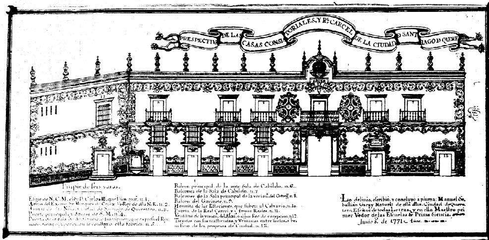
Proyecto de la fachada del Palacio Municipal de Querétaro. AGI, Mapas y Planos, México, 600
