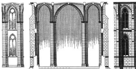
3. Sección transversal de la iglesia de Santa Isabel de Marburgo (Jantzen)
