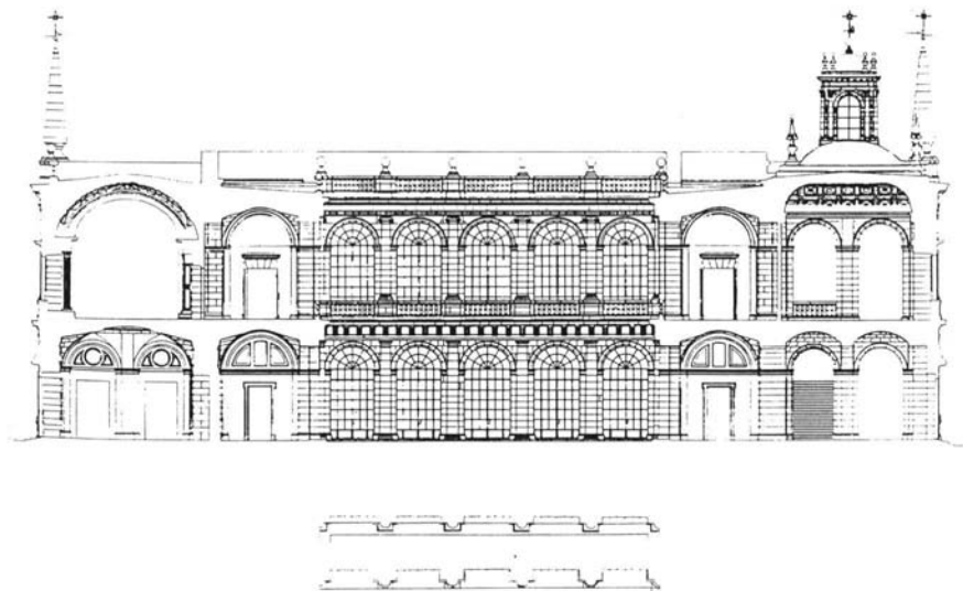
CASA LONJA. Sección F. Villanueva
