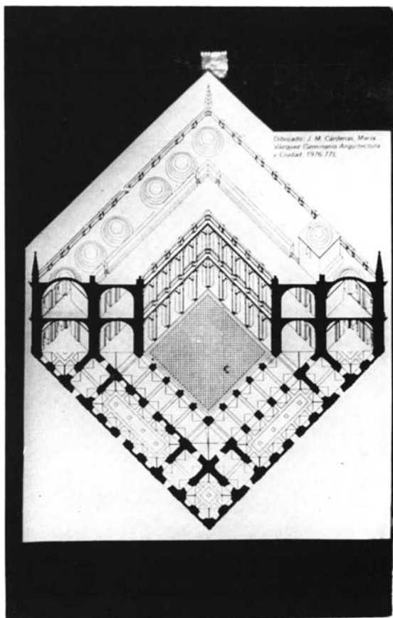
Casa Lonja de Sevilla. Planta y sección en perspectiva. (Dibujo de J. M. Cárdenas y María Vázquez. Semin. Arq. y Ciudad 1976-77).
